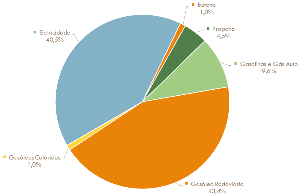
Figura 58 - Emissões de CO 2 por Vetor Energético Consumido em 2030 [%]
