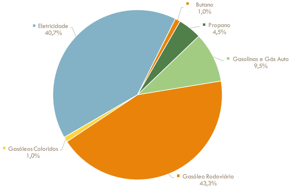
Figura 57 - Emissões de CO 2 por Vetor Energético Consumido em 2020 [%]
