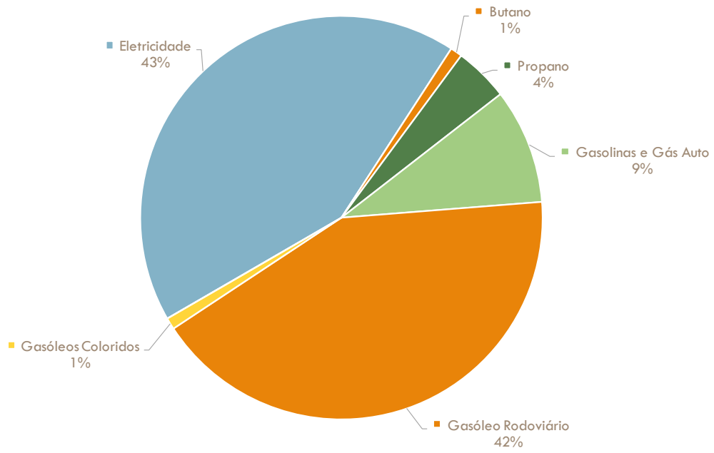
Figura 59 - Emissões de CO 2 por Vetor Energético Consumido em 2050 [%]
