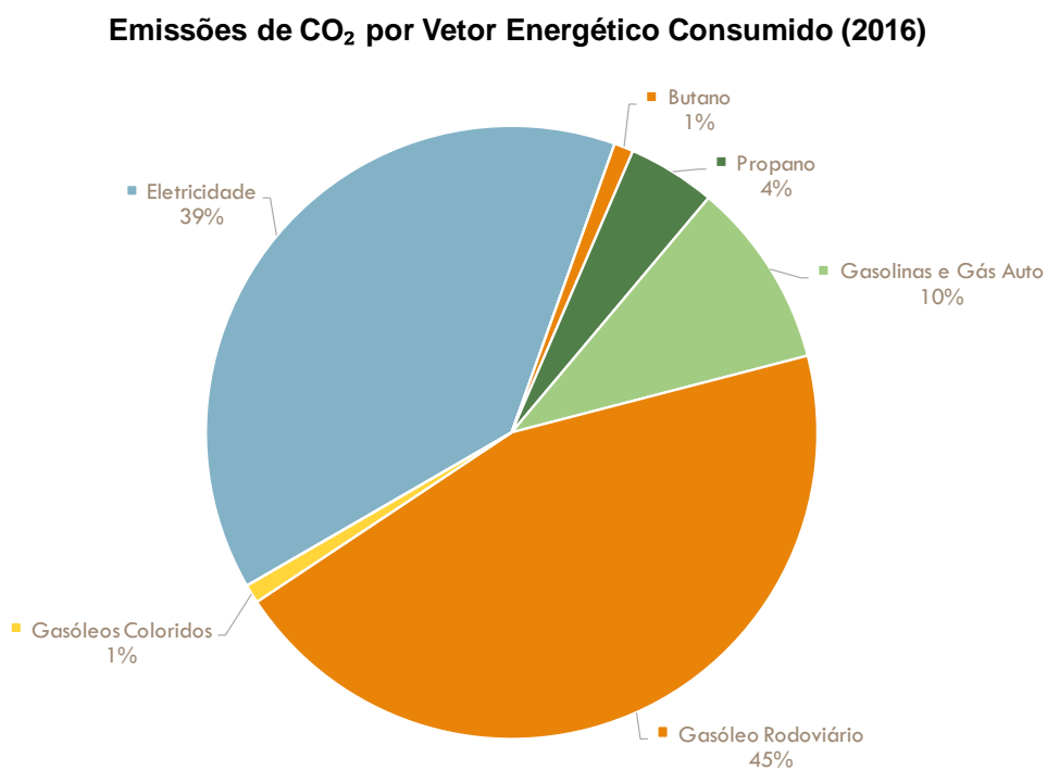
Figura 56 - Emissões de CO 2 por Vetor Energético Consumido em 2016 [%]
