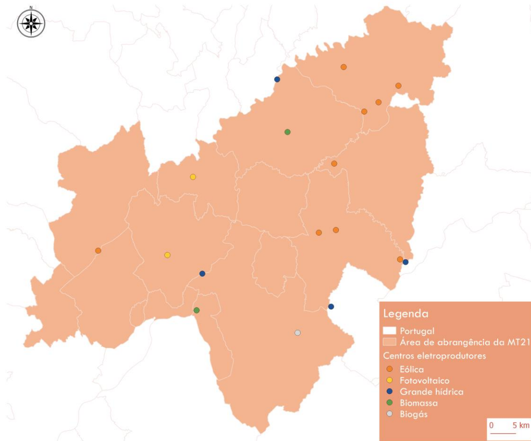
Figura 63 - Centros electroprodutores de base renovável localizados na região de abrangência da MédioTejo21 (adaptado de INEGI, 2017)
