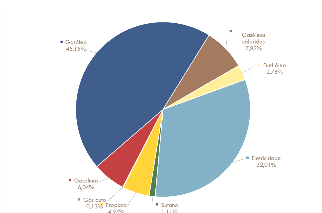
Figura 37: Emissões de CO 2 no município de Ferreira do Zêzere por vetor energético [%]
