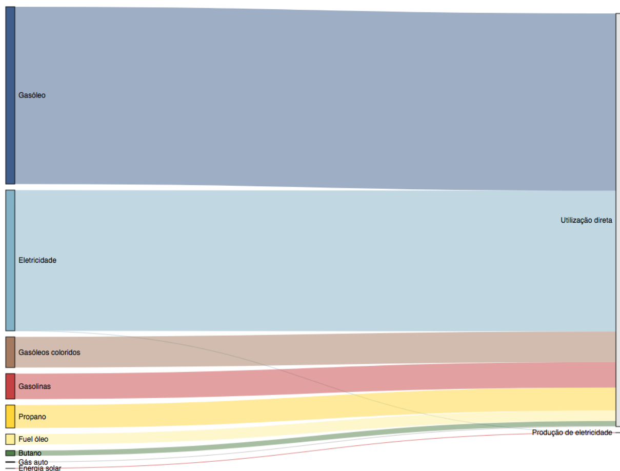
Figura 35: Diagrama de Sankey da utilização de fontes de energia primária no município de Ferreira do Zêzere
