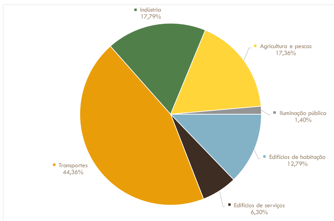
Figura 39: Emissões de CO 2 no município de Ferreira do Zêzere por setor consumidor de energia [%]
