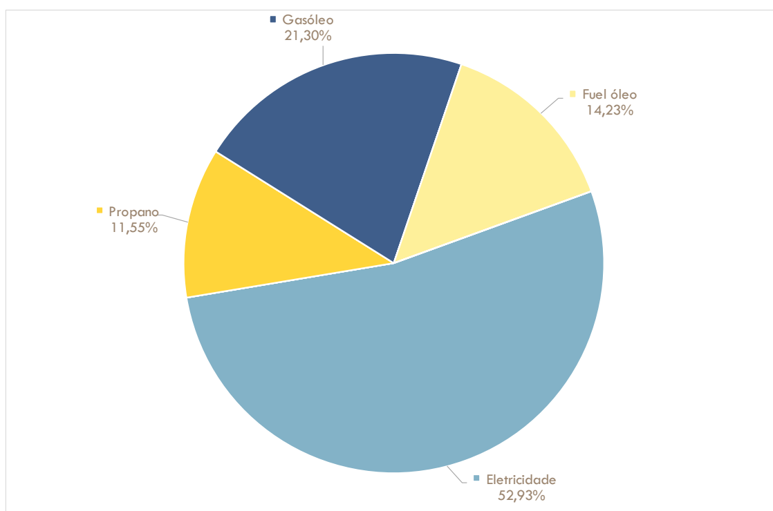
Figura 58: Utilização de energia final na indústria transformadora no município de Ferreira do Zêzere por vetor energético [%]
