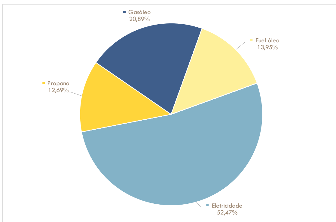
Figura 52: Utilização de energia final na indústria no município de Ferreira do Zêzere por vetor energético [%]
