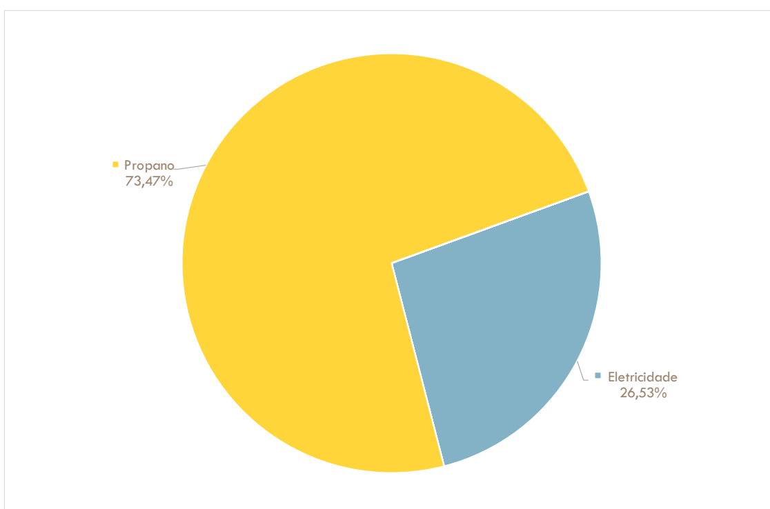
Figura 63: Emissões de CO2 no subsetor construção e obras públicas no município de Ferreira do Zêzere por vetor energético [%]
