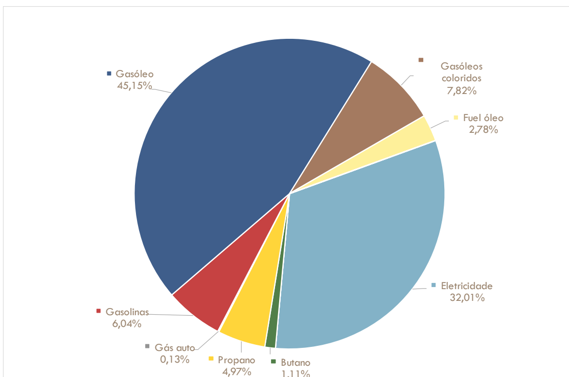
Figura 34: Emissões de CO 2 no município de Ferreira do Zêzere por vetor energético primário [%]
