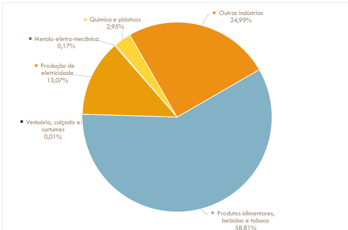
Figura 58: Utilização de energia final na indústria transformadora no município de Mação por agrupamento de atividade económica [%]
