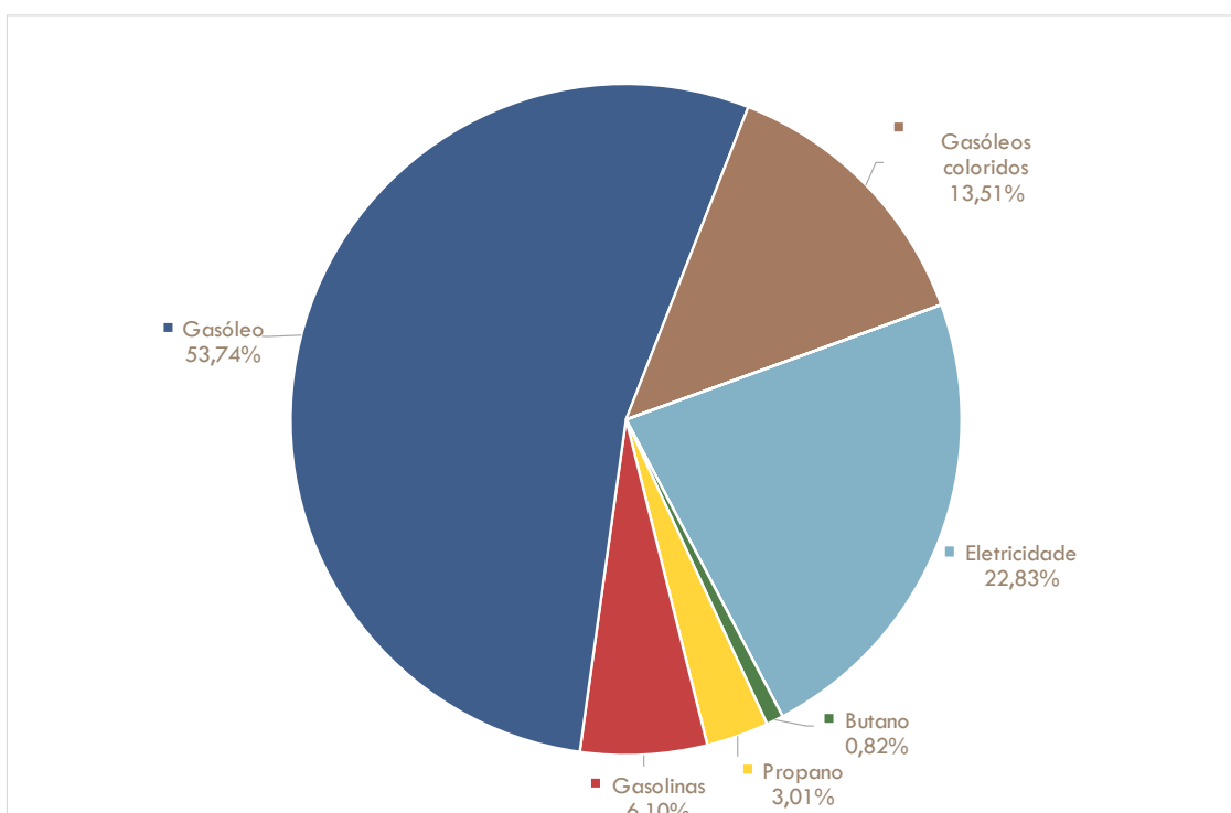
Figura 37: Emissões de CO 2 no município de Mação por vetor energético [%]
