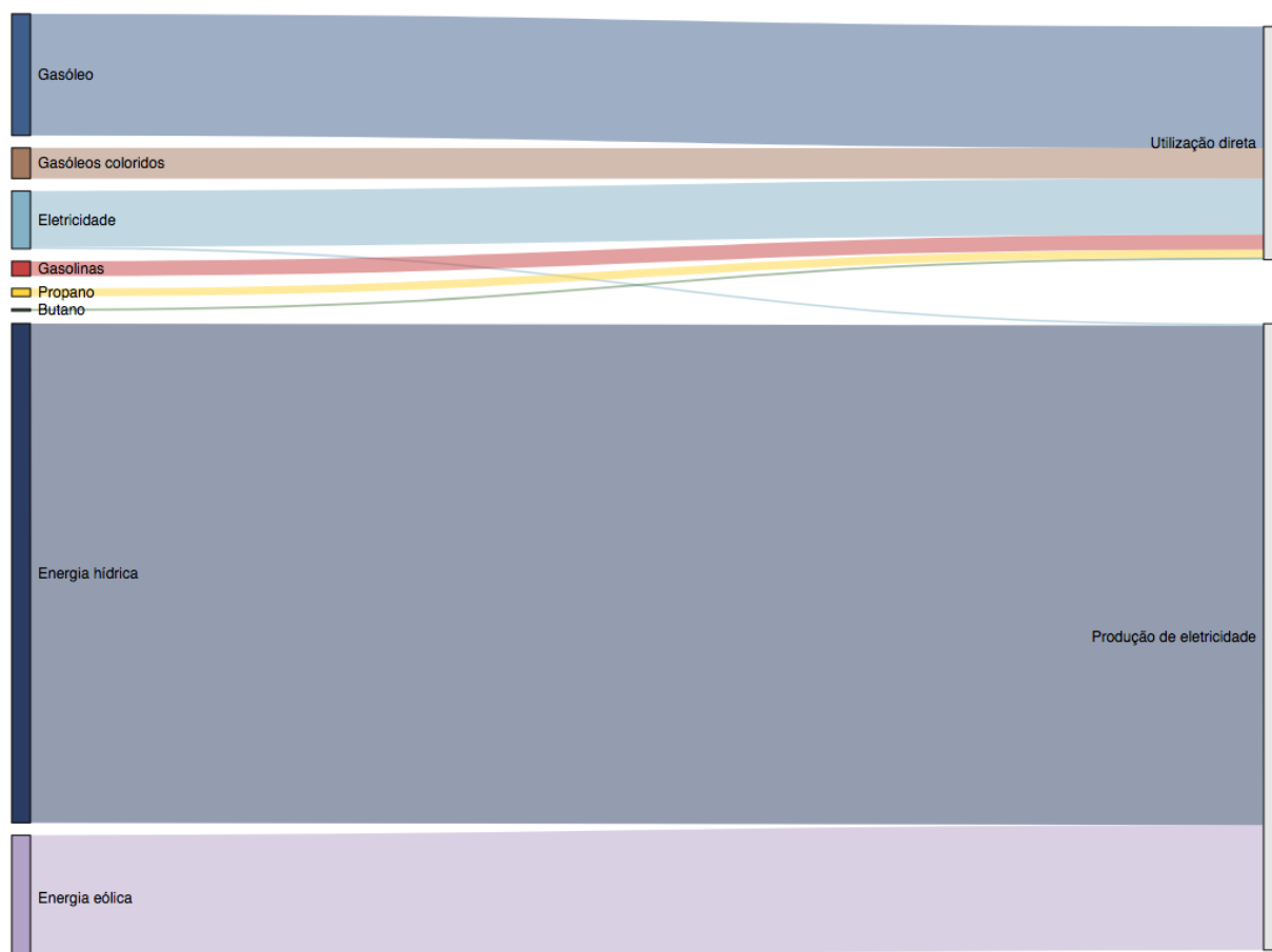
Figura 35: Diagrama de Sankey da utilização de fontes de energia primária no município de Mação
