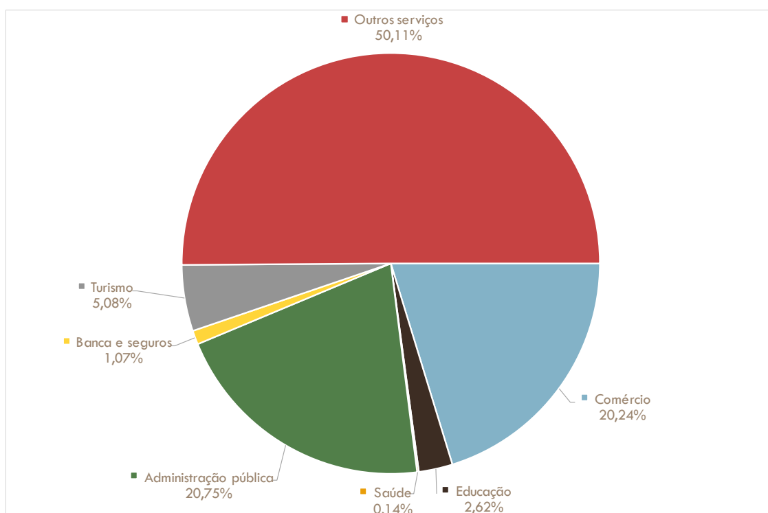
Figura 45: Emissões de CO 2 em serviços no município de Mação por agrupamento de atividade económica [%]
