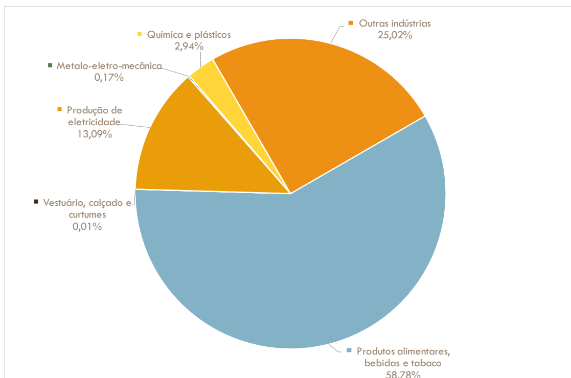
Figura 59: Emissões de CO 2 na indústria transformadora no município de Mação por agrupamento de atividade económica [%]
