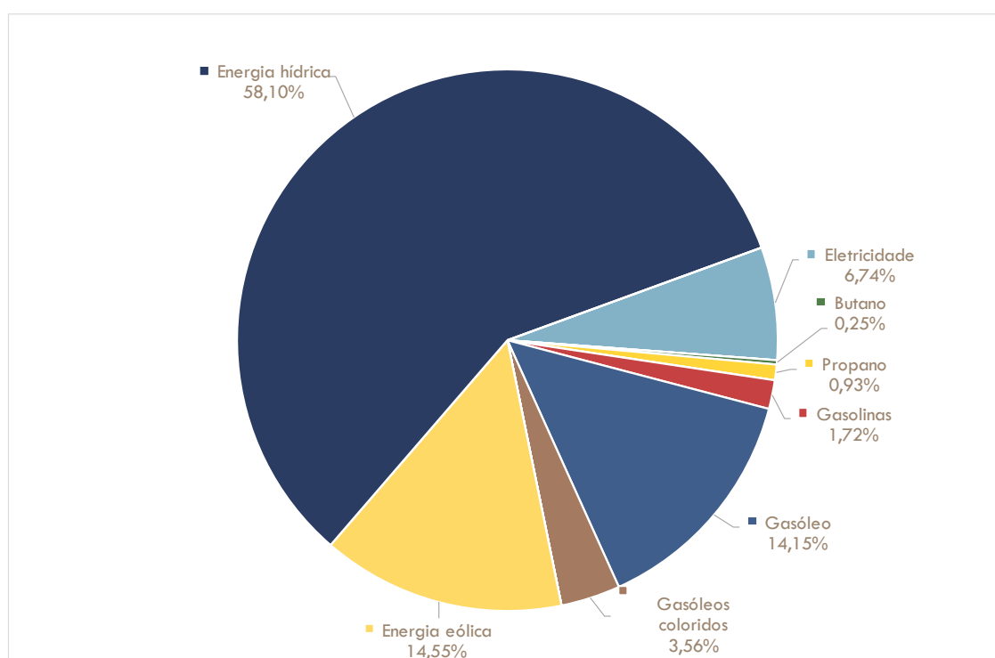
Figura 33: Consumo total de energia primária no município de Mação por vetor energético [%]
