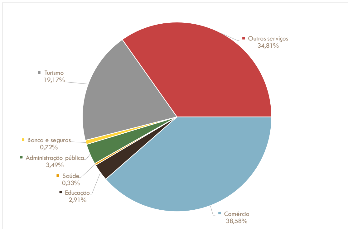
Figura 44: Utilização de energia final em serviços no município de Ourém por agrupamento de atividade económica [%]
