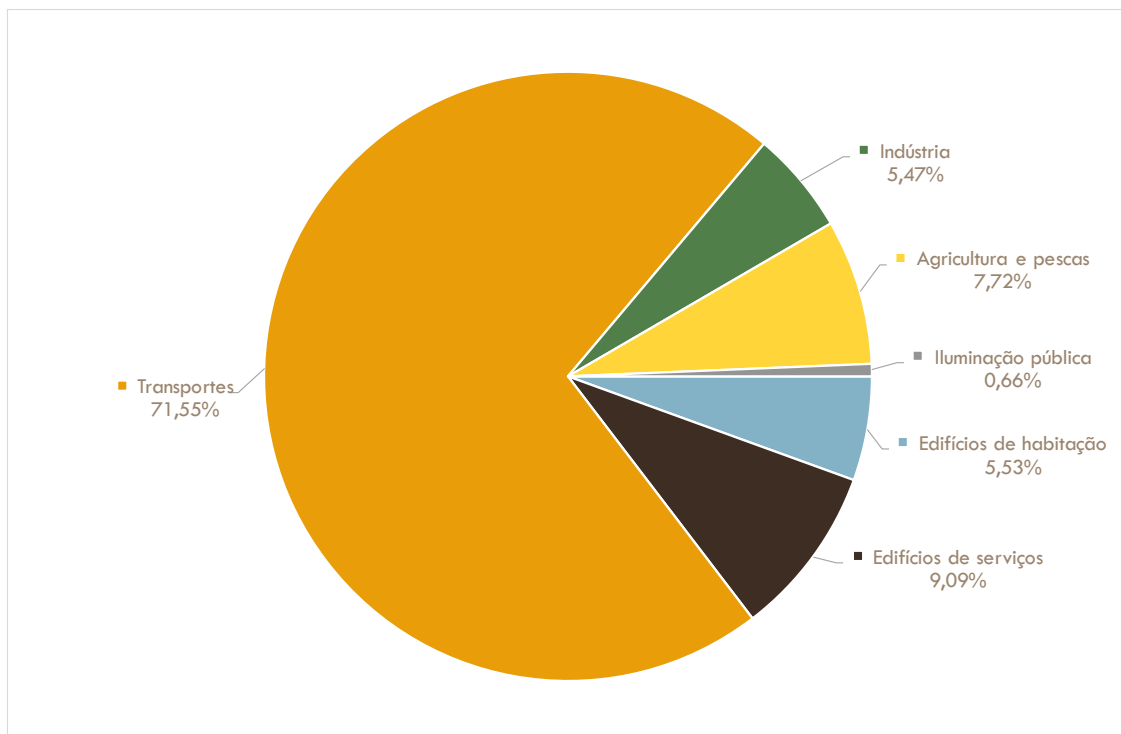
Figura 39: Emissões de CO 2 no município de Ourém por setor consumidor de energia [%]
