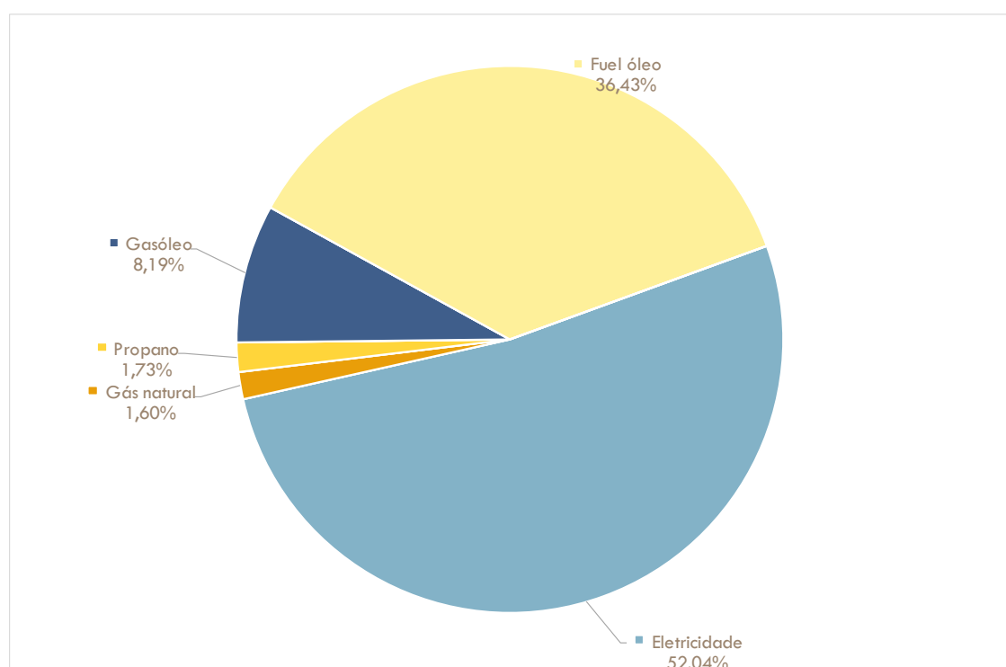
Figura 59: Emissões de CO 2 na indústria transformadora no município de Ourém por vetor energético [%]
