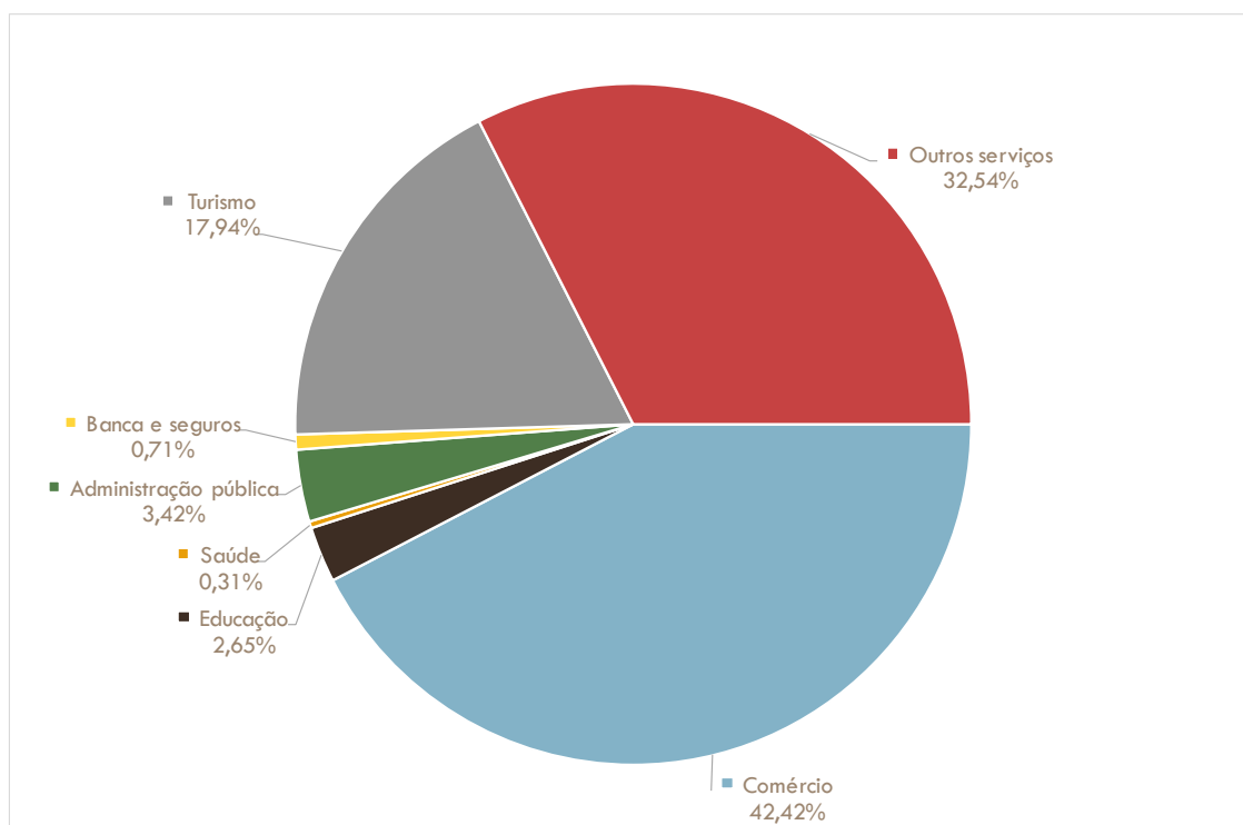
Figura 45: Emissões de CO 2 em serviços no município de Ourém por agrupamento de atividade económica [%]
