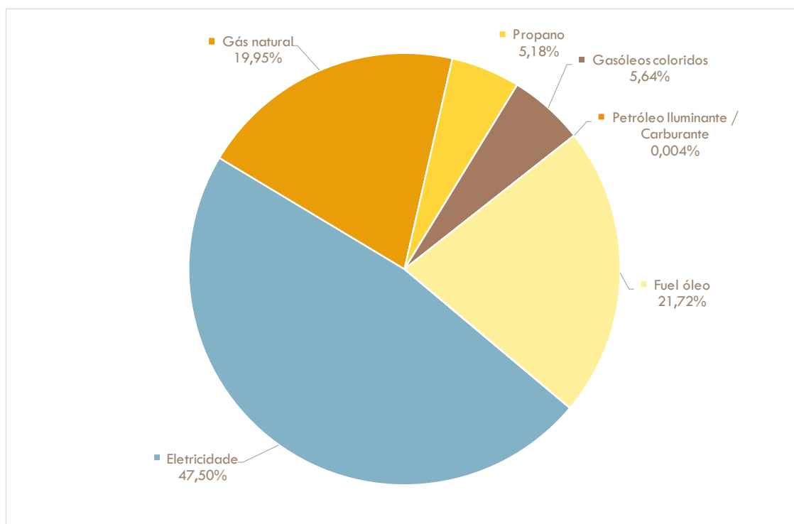
Figura 42: Utilização de energia final no setor de serviços no município de Ourém por vetor energético [%]
