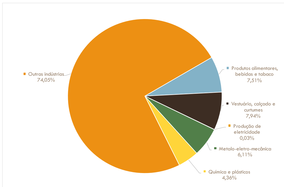
Figura 60: Utilização de energia final na indústria transformadora no município de Ourém por agrupamento de atividade económica [%]
