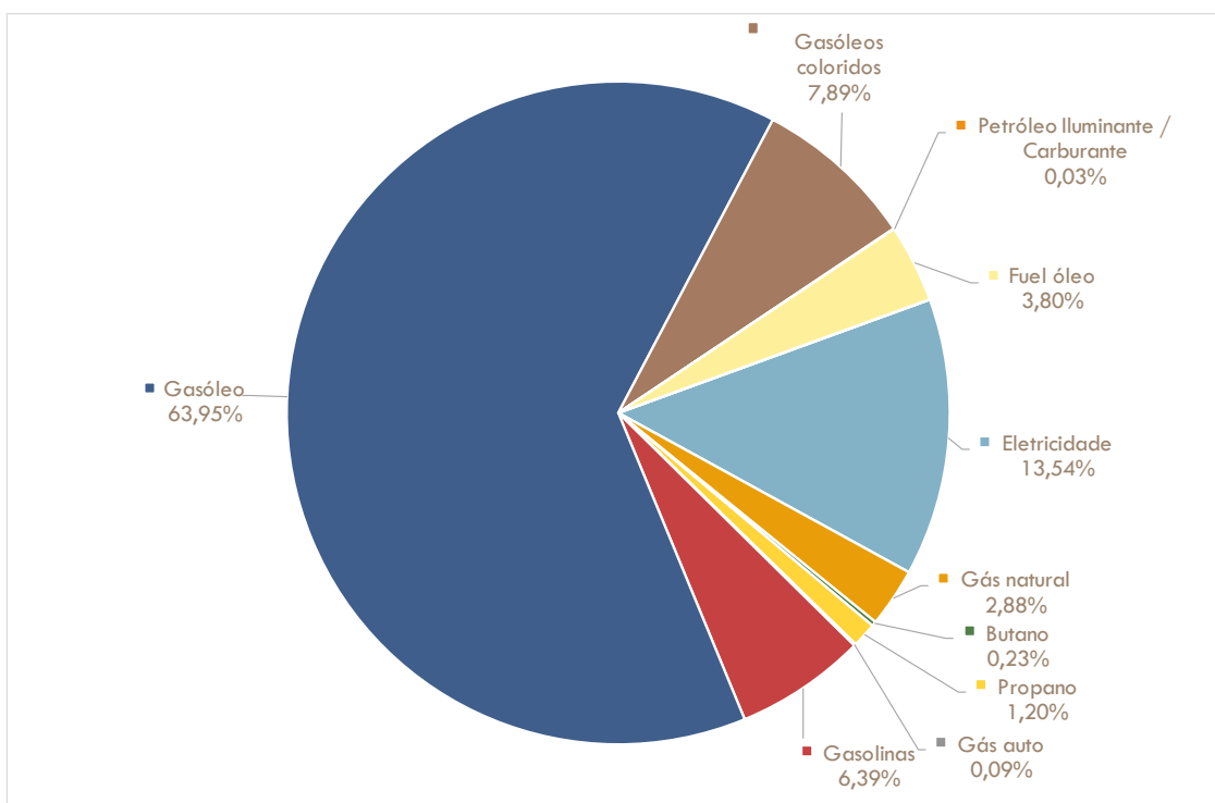
Figura 36: Utilização de energia final no município de Ourém por vetor energético [%]
