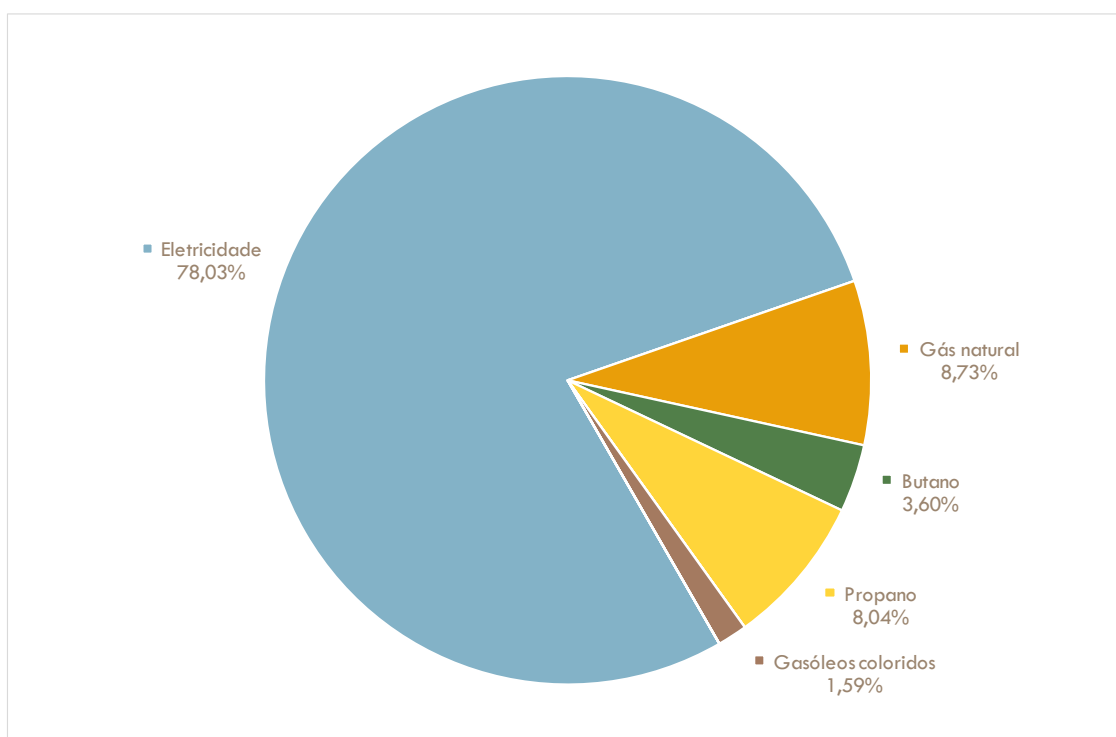
Figura 41: Emissões de CO 2 no setor residencial no município de Ourém por vetor energético [%]
