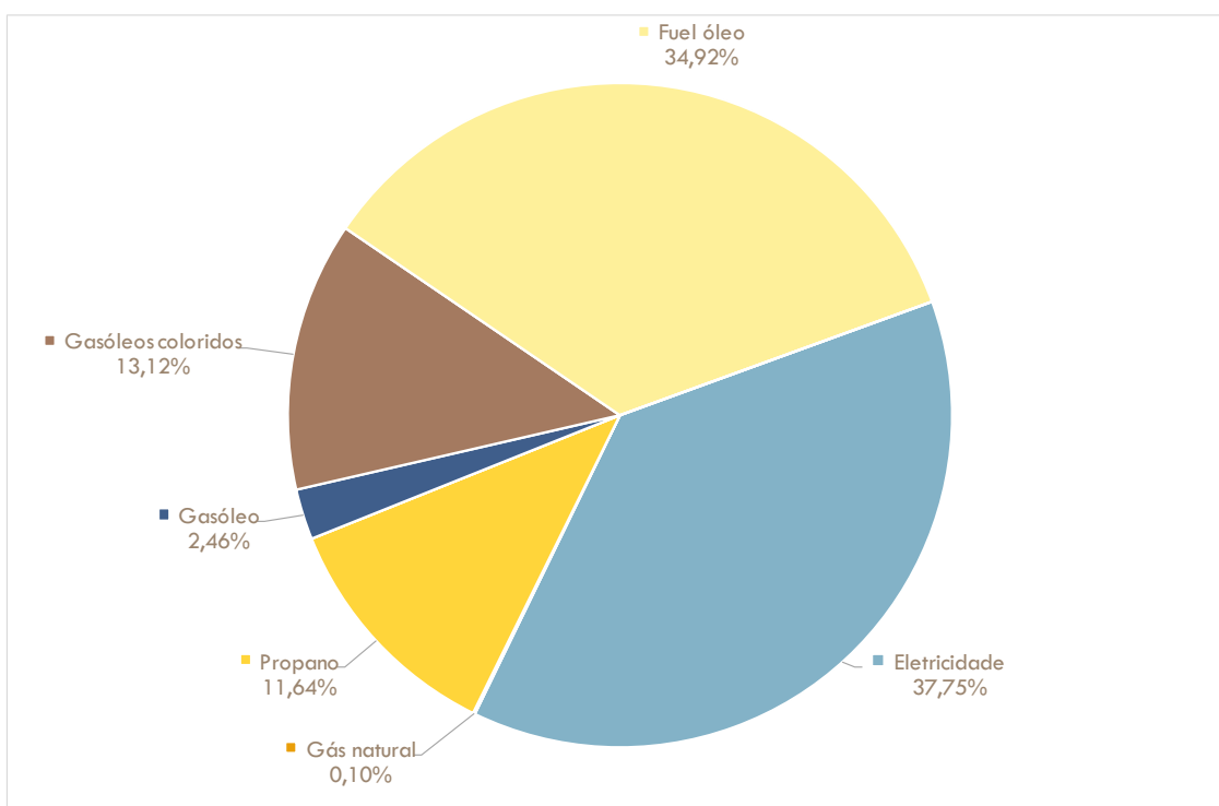
Figura 63: Emissões de CO 2 no subsetor construção e obras públicas no município de Ourém por vetor energético [%]
