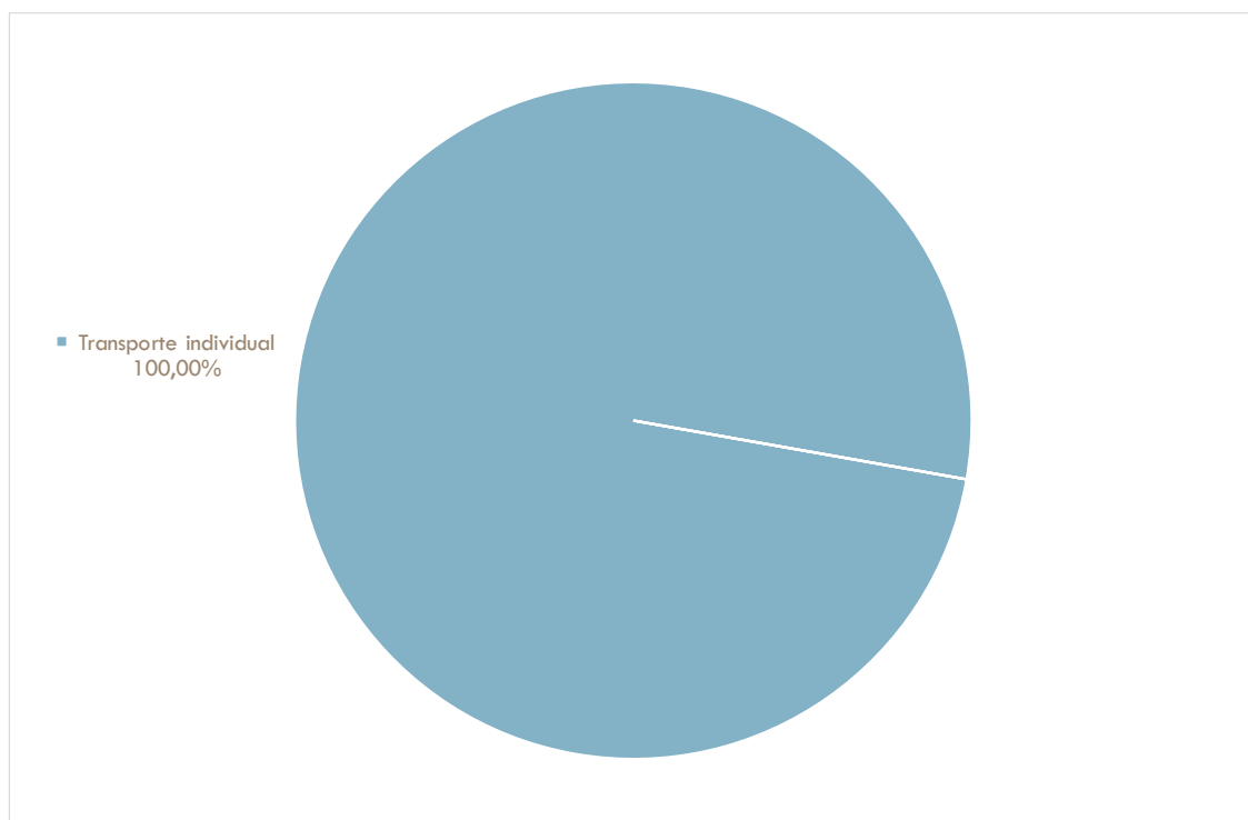
Figura 50: Utilização de energia final no subsetor transportes privados no município de Ourém por modo de transporte [%]
