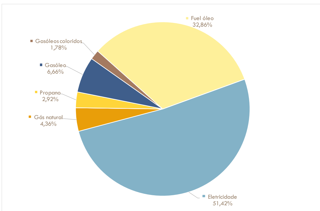
Figura 53: Emissões de CO 2 na indústria no município de Ourém por vetor energético [%]
