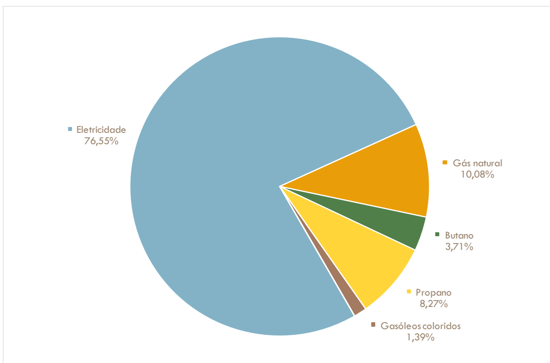
Figura 40: Utilização de energia final no setor residencial no município de Ourém por vetor energético [%]
