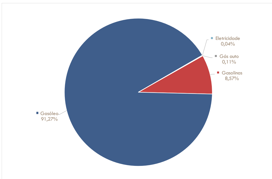
Figura 47: Emissões de CO 2 no setor dos transportes no município de Ourém por vetor energético [%]
