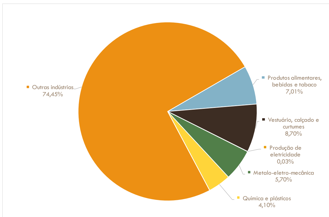
Figura 61: Emissões de CO 2 na indústria transformadora no município de Ourém por agrupamento de atividade económica [%]
