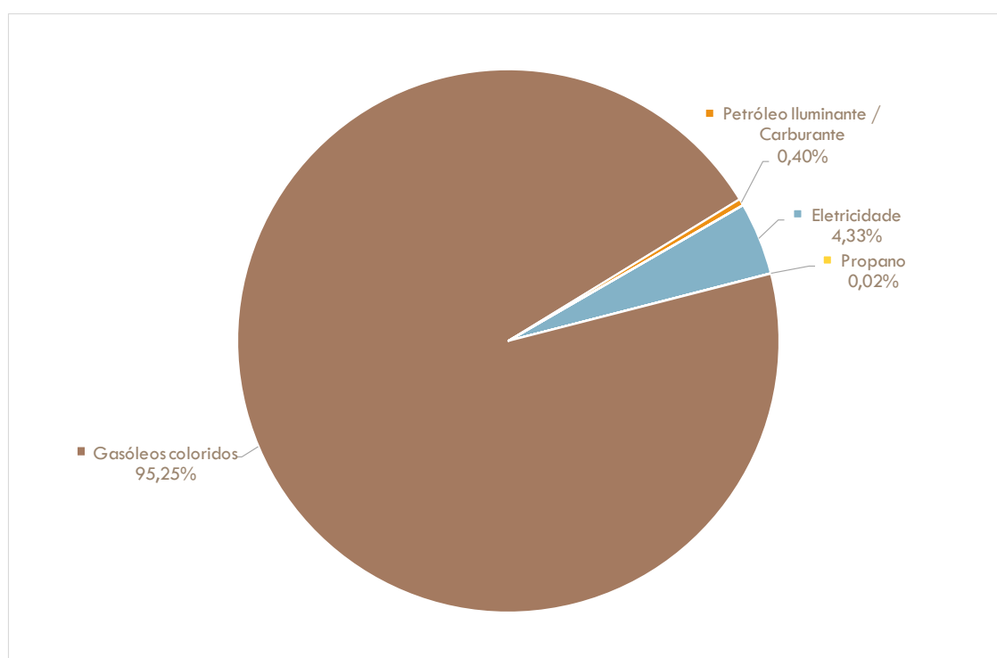
Figura 65: Emissões de CO 2 no setor da agricultura e pescas no município de Ourém por vetor energético [%]
