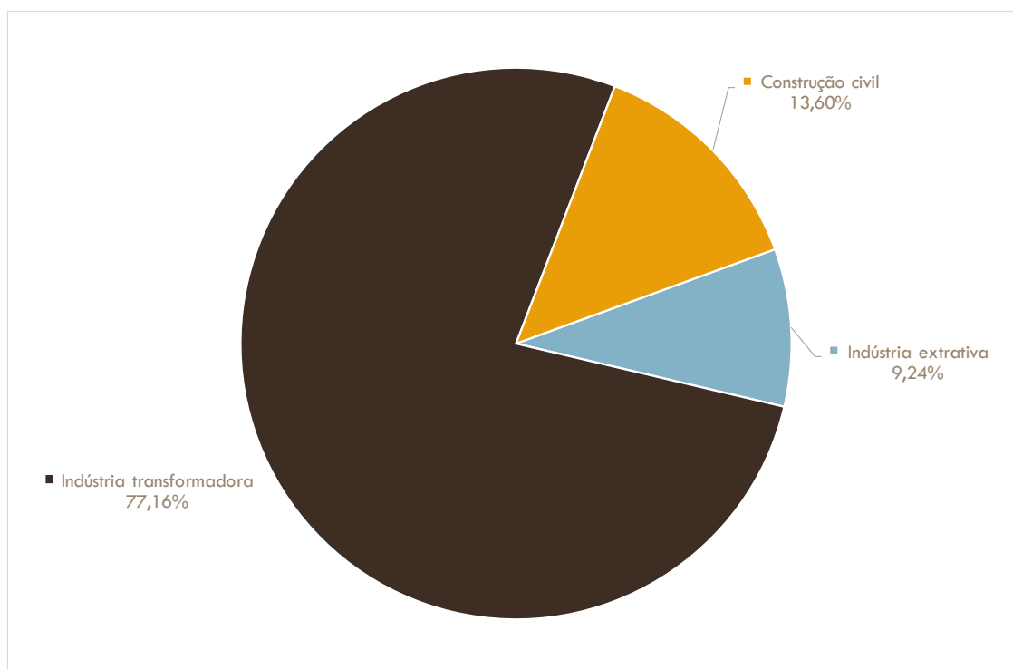
Figura 55: Emissões de CO 2 na indústria no município de Ourém por subsetor de atividade [%]
