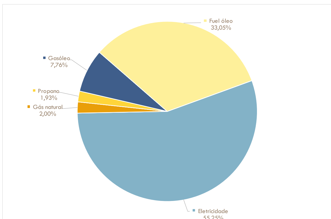
Figura 58: Utilização de energia final na indústria transformadora no município de Ourém por vetor energético [%]
