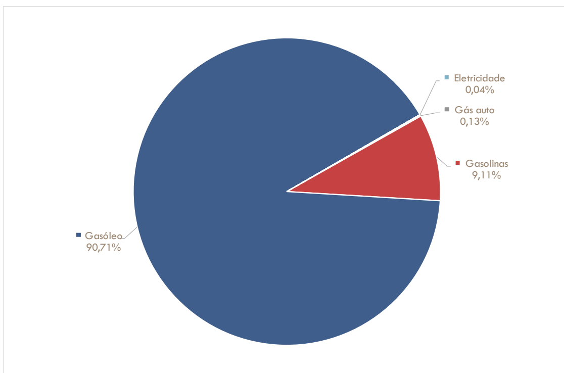
Figura 48: Utilização de energia final no subsetor transportes privados no município de Ourém por vetor energético [%]
