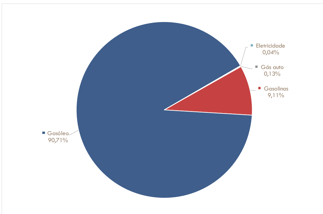
Figura 46: Utilização de energia final no setor dos transportes no município de Ourém por vetor energético [%]
