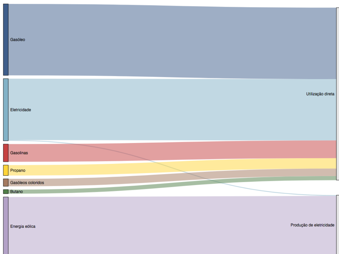
Figura 35: Diagrama de Sankey da utilização de fontes de energia primária no município de Proença-a-nova
